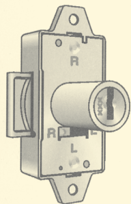
Drehstangenschloss mit Wechselzylinder Espagnolette lock with alternating cylinder Serrure espagnolette avec cylindre variable
